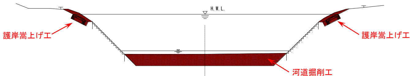
横断面図(井戸坂橋上流付近)
