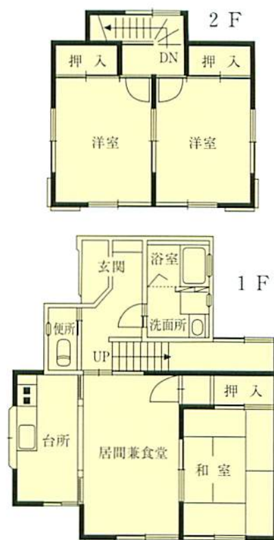
〈平面図〉
